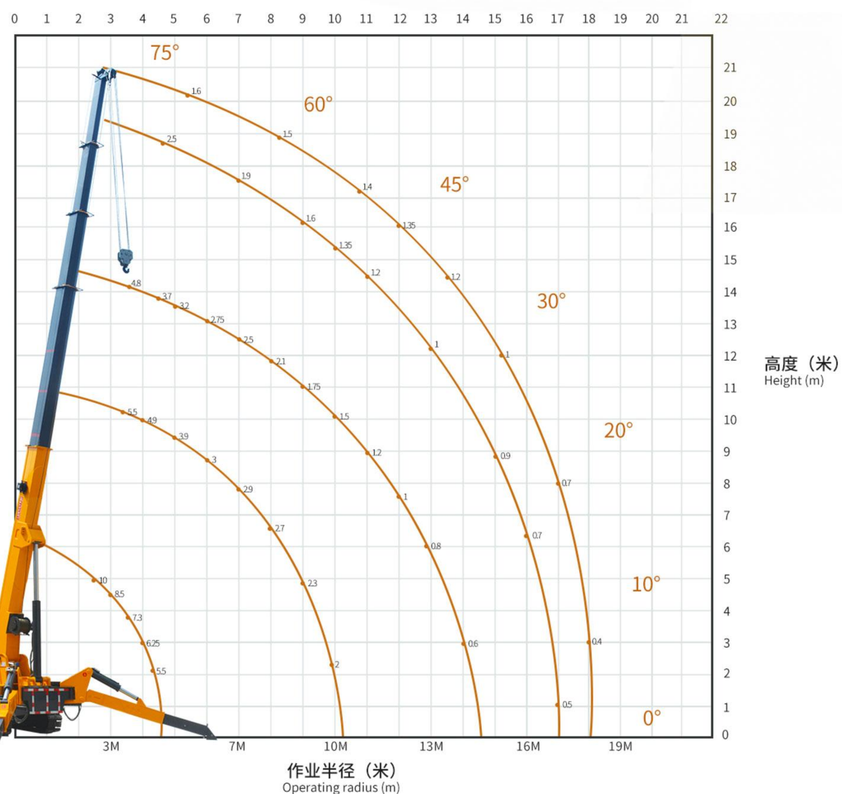
10吨蜘蛛吊机吊重表 10 ton spider crane lifting weight chart
