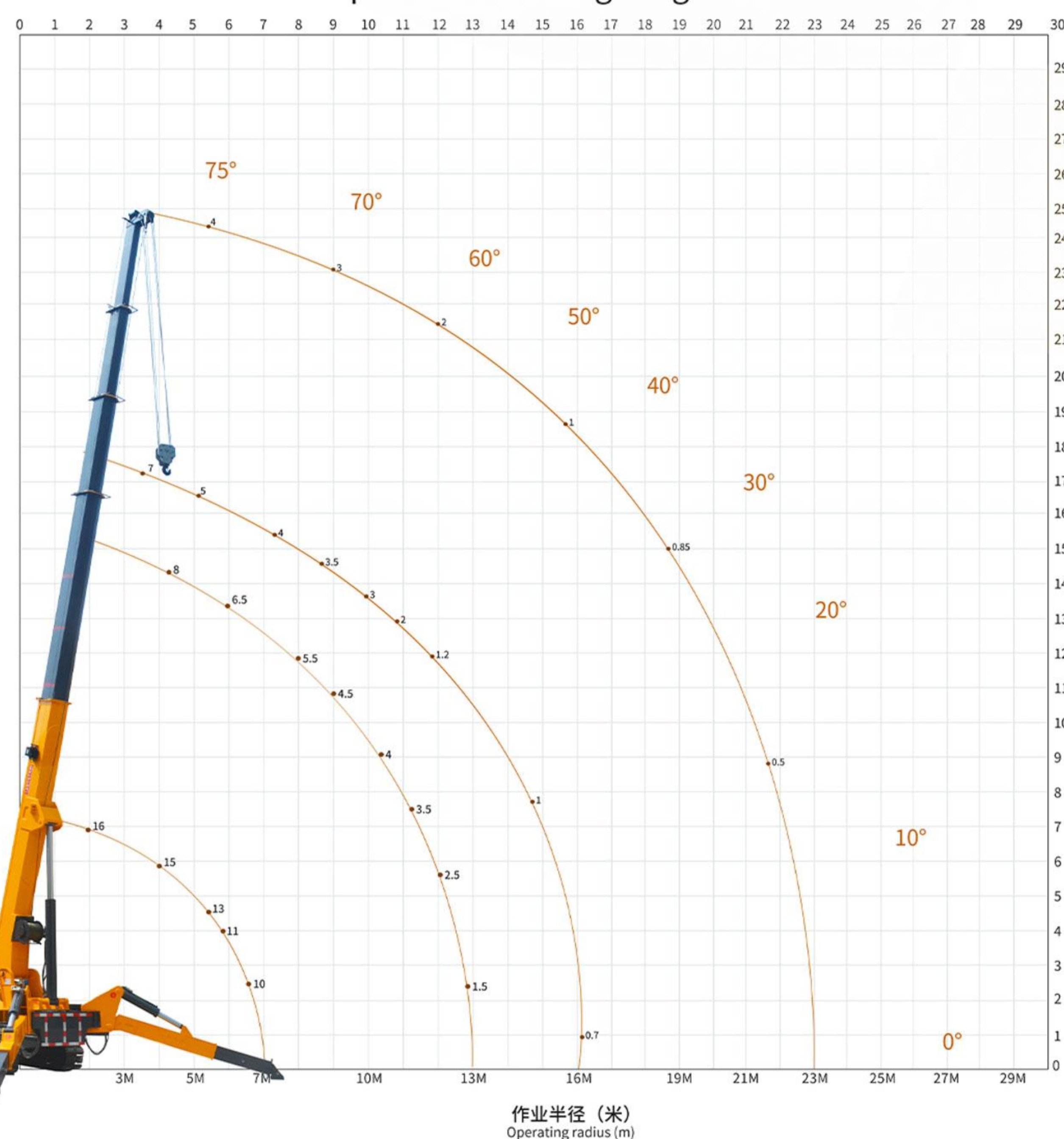
16吨蜘蛛吊机吊重表 16 ton spider crane lifting weight chart
