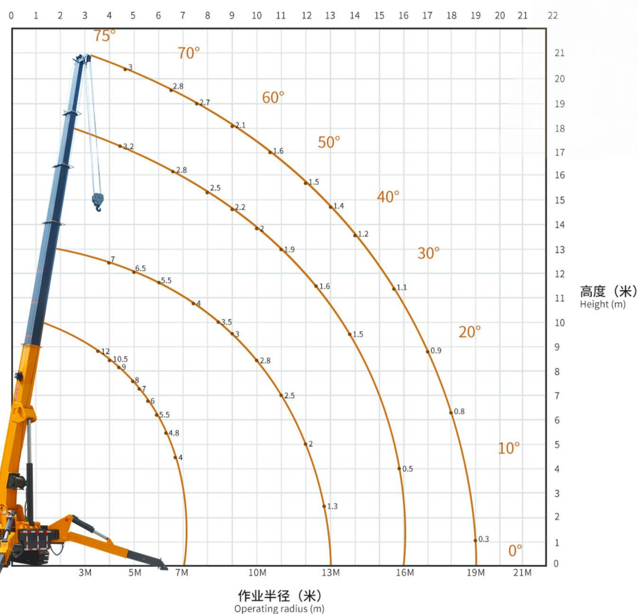
12吨蜘蛛吊机吊重表 12 ton spider crane lifting weight chart
