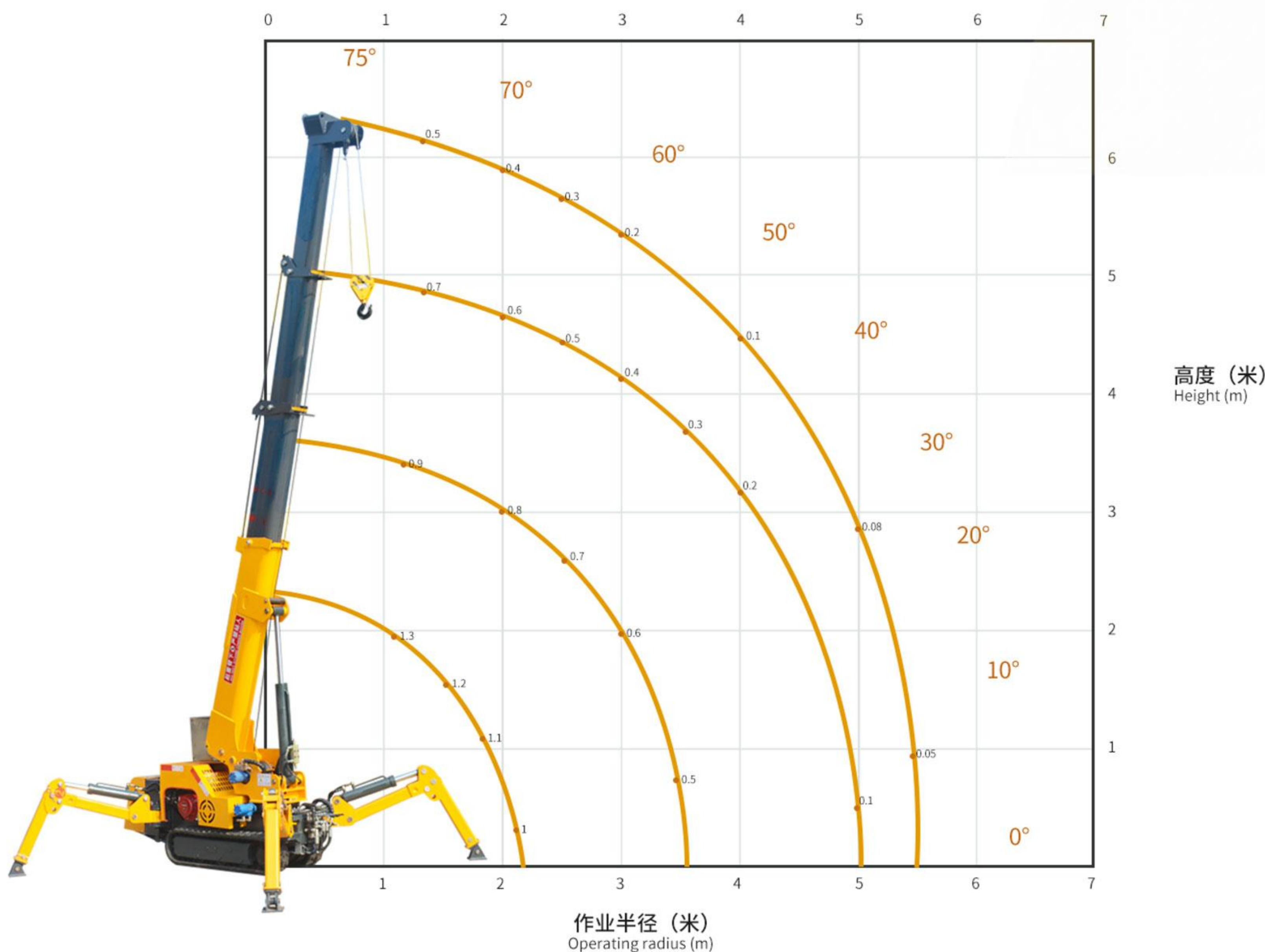
1.2吨蜘蛛吊吊重表 1.2 ton spider crane lifting weight chart
